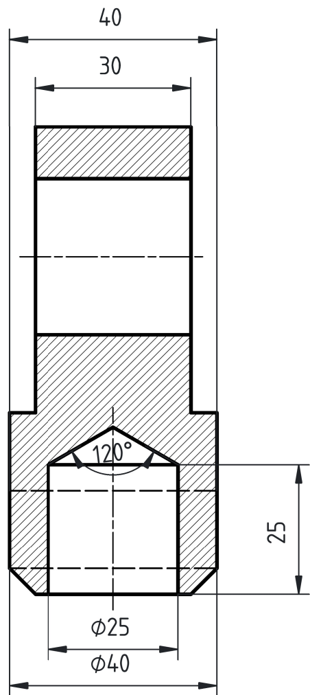
Coupe AA
