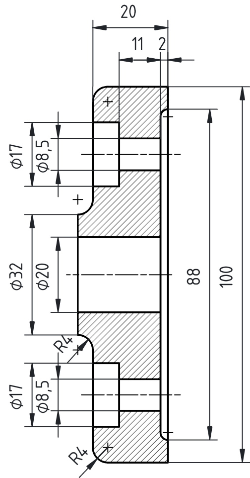
Coupe AA
