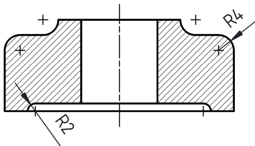
Coupe BB
