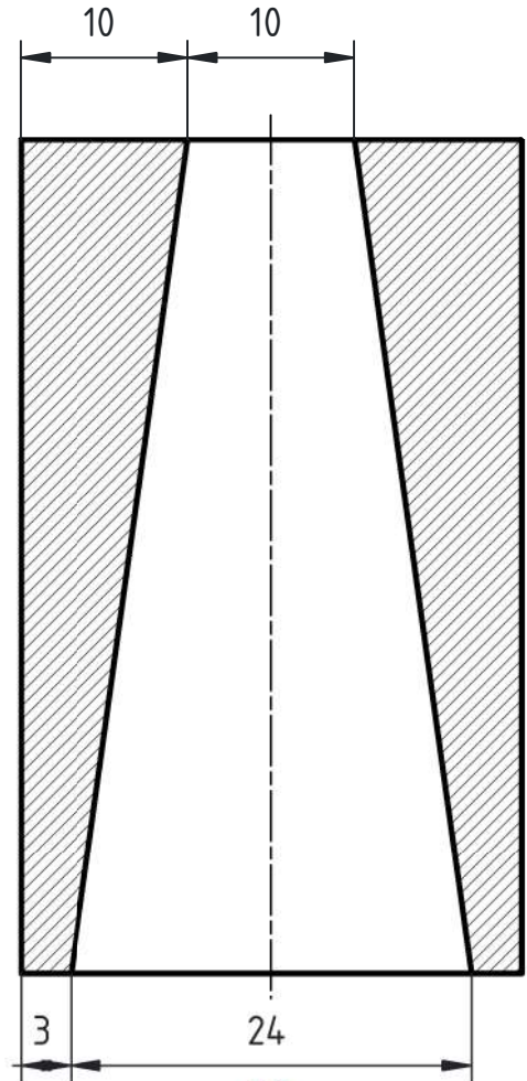
Coupe BB
