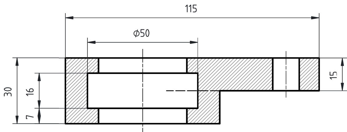
Coupe AA
