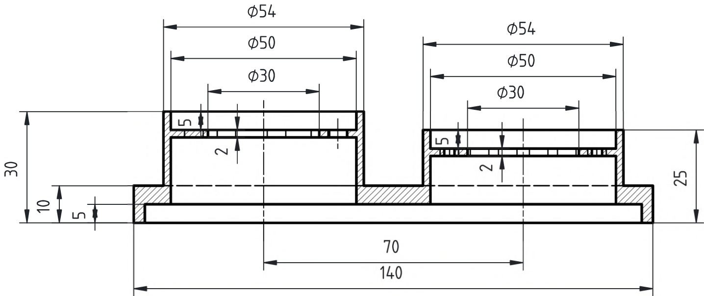
Coupe AA
