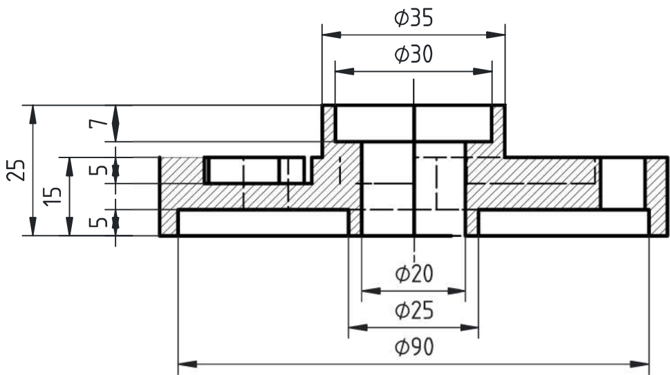
Coupe AA
