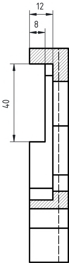
Coupe AA
