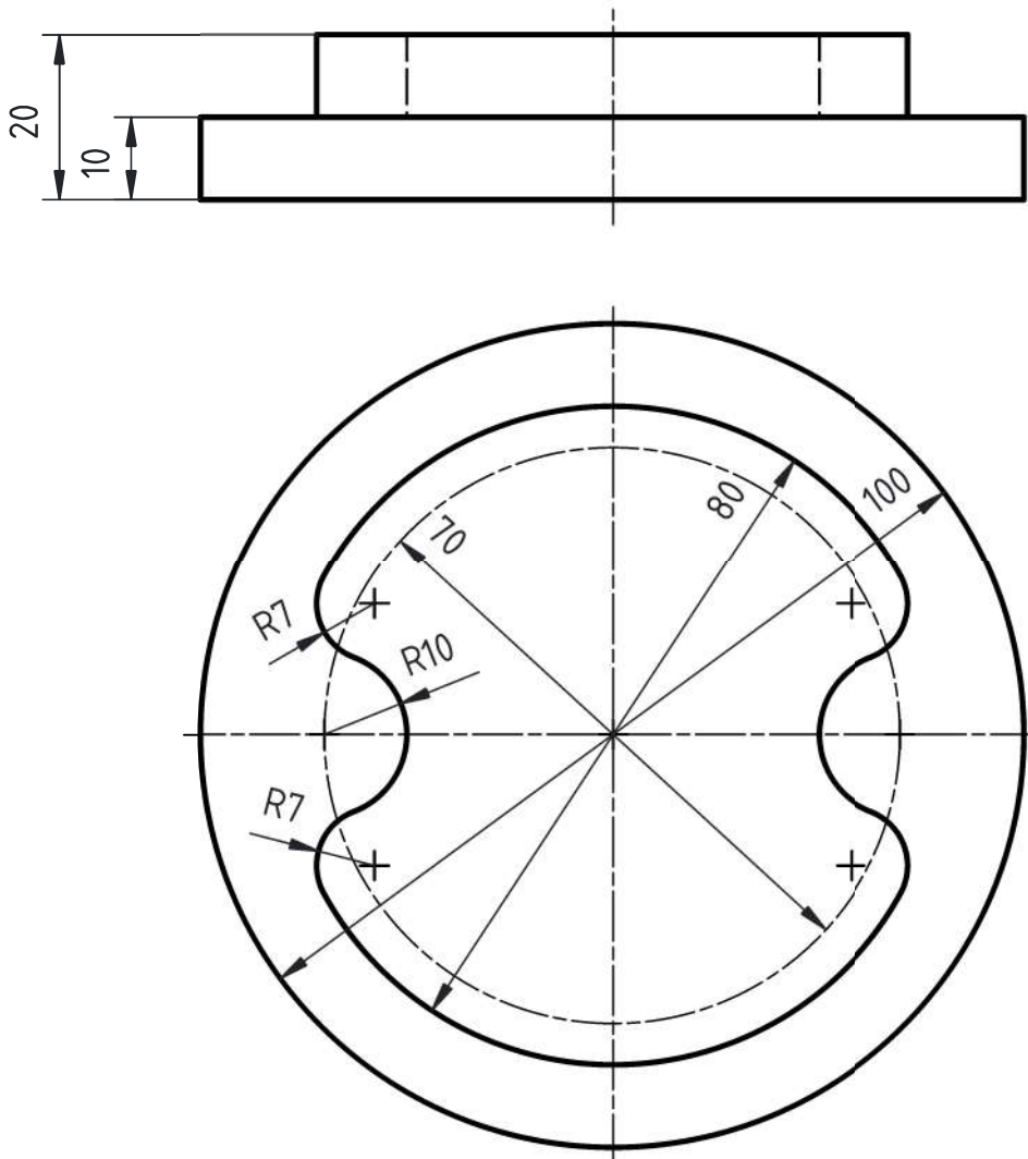
Pièce mâle
