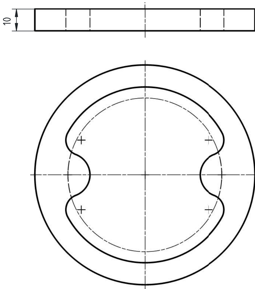
Pièce femelle
