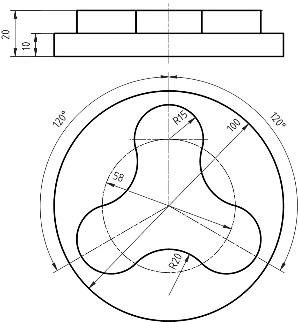
Pièce mâle
