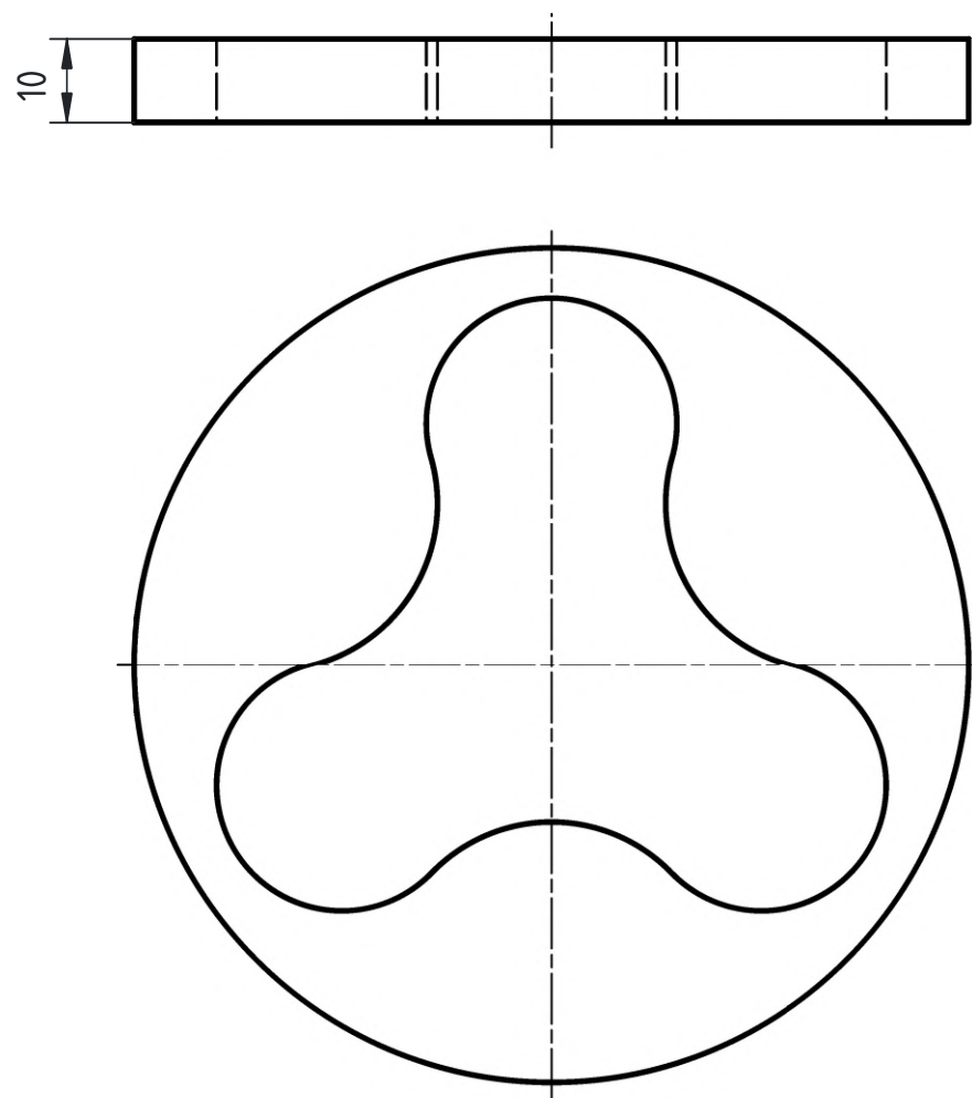
Pièce femelle
