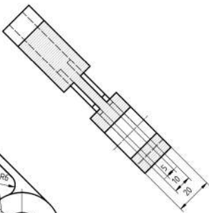
Coupe BB
