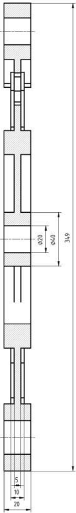
Coupe AA
