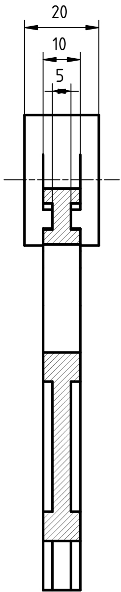
Coupe BB
