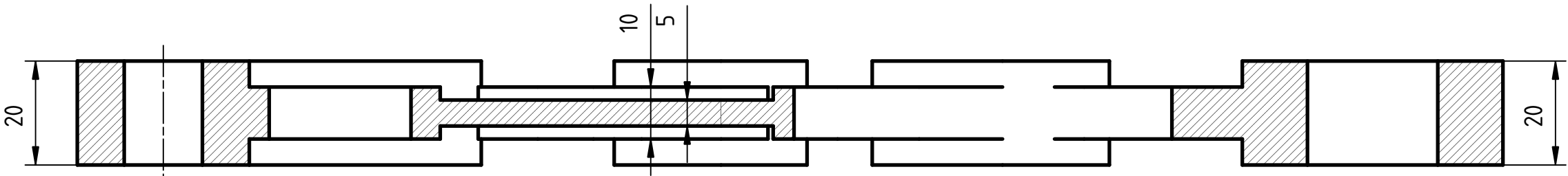
Coupe AA
