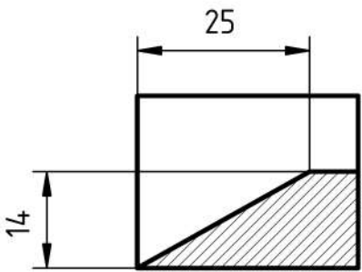
Coupe AA
