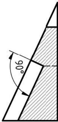
Coupe AA
