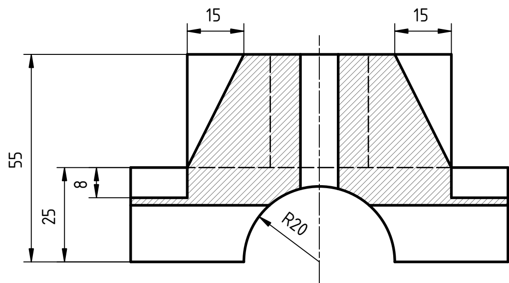
Coupe AA
