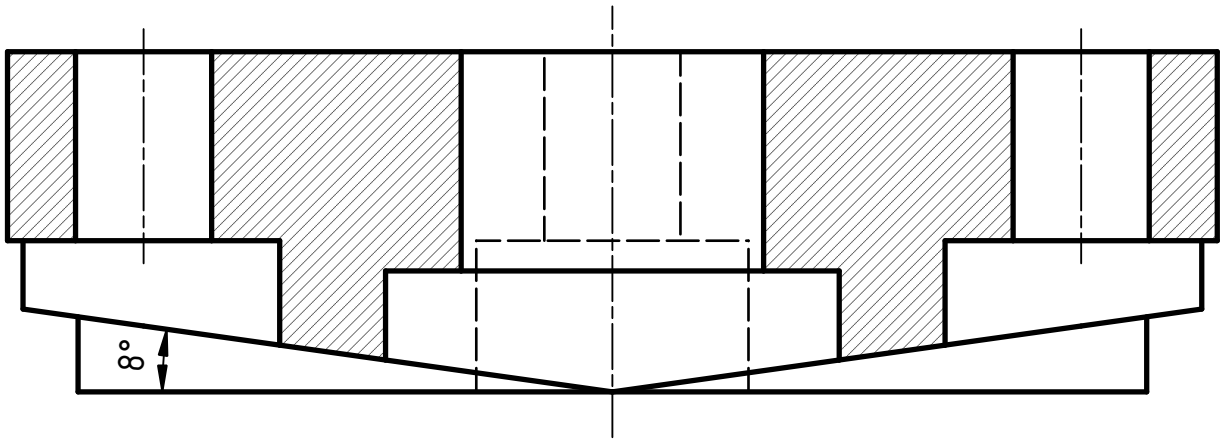
Coupe BB
