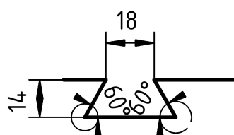
Vue suivant A
