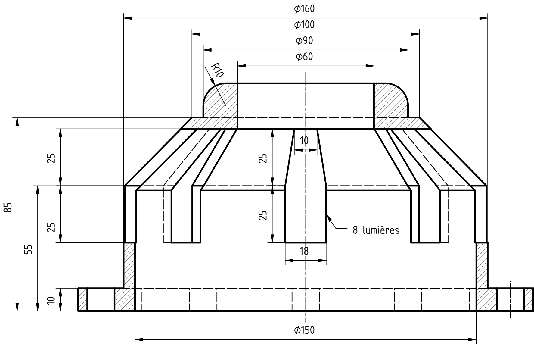
Coupe AA
