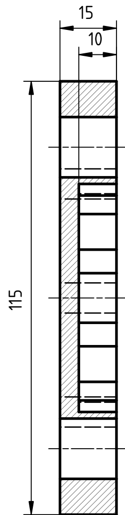
Coupe AA
